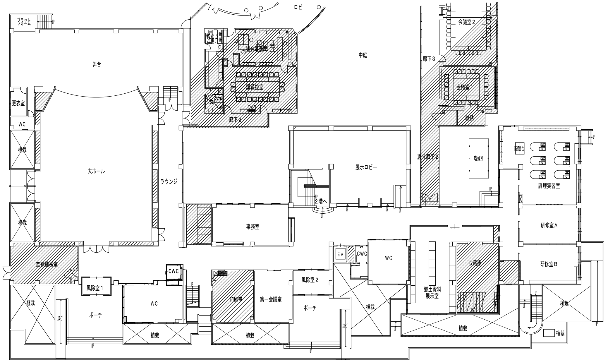
東庄町公民館1階平面図
