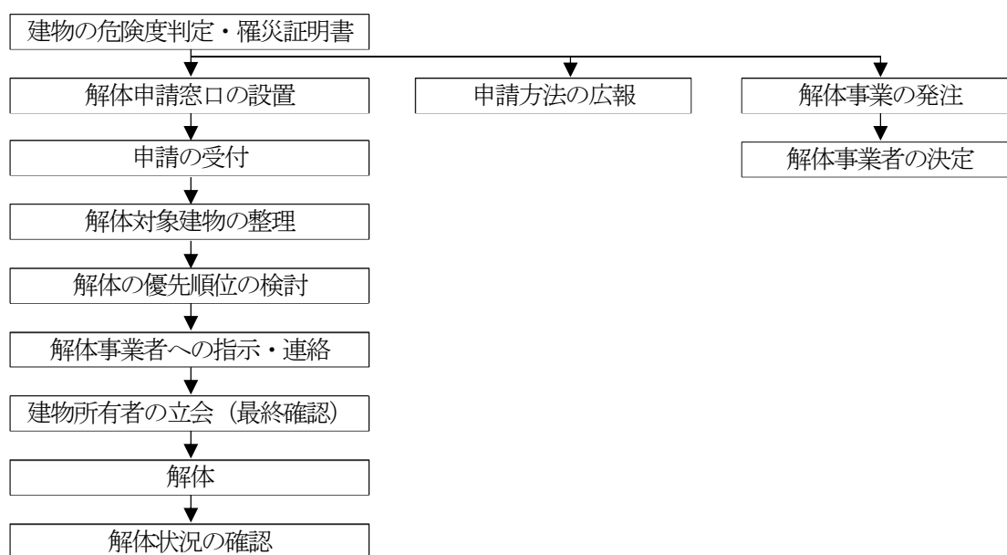
図表3-2 東庄町が実施する解体・撤去の手順
