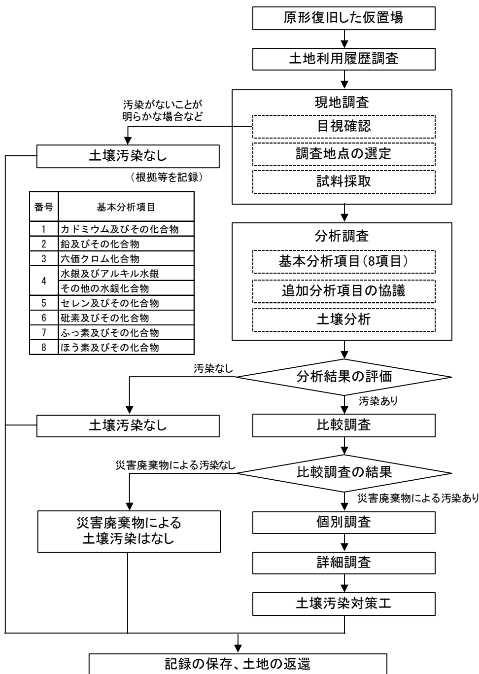
図表6.6 災害廃棄物仮置場返還に伴う手順
