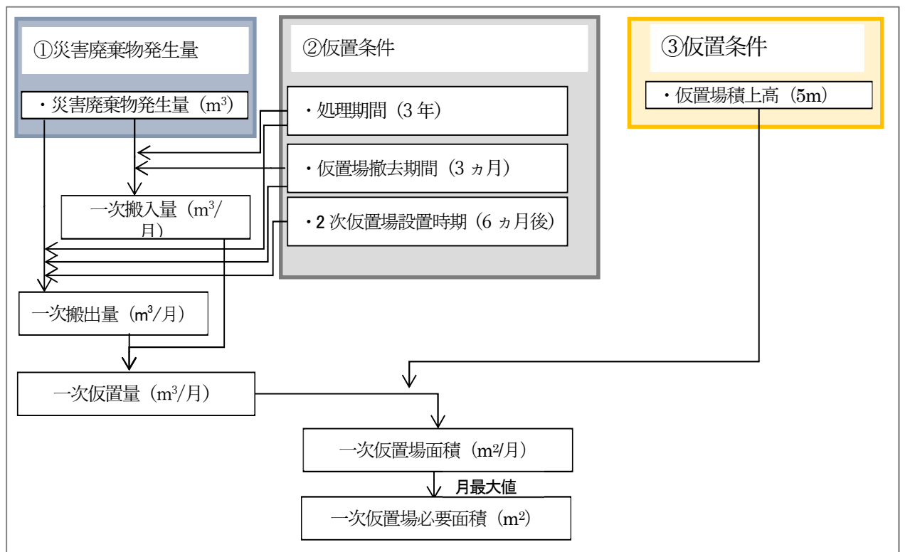
図表2.6 仮置場必要面積の計算方法
