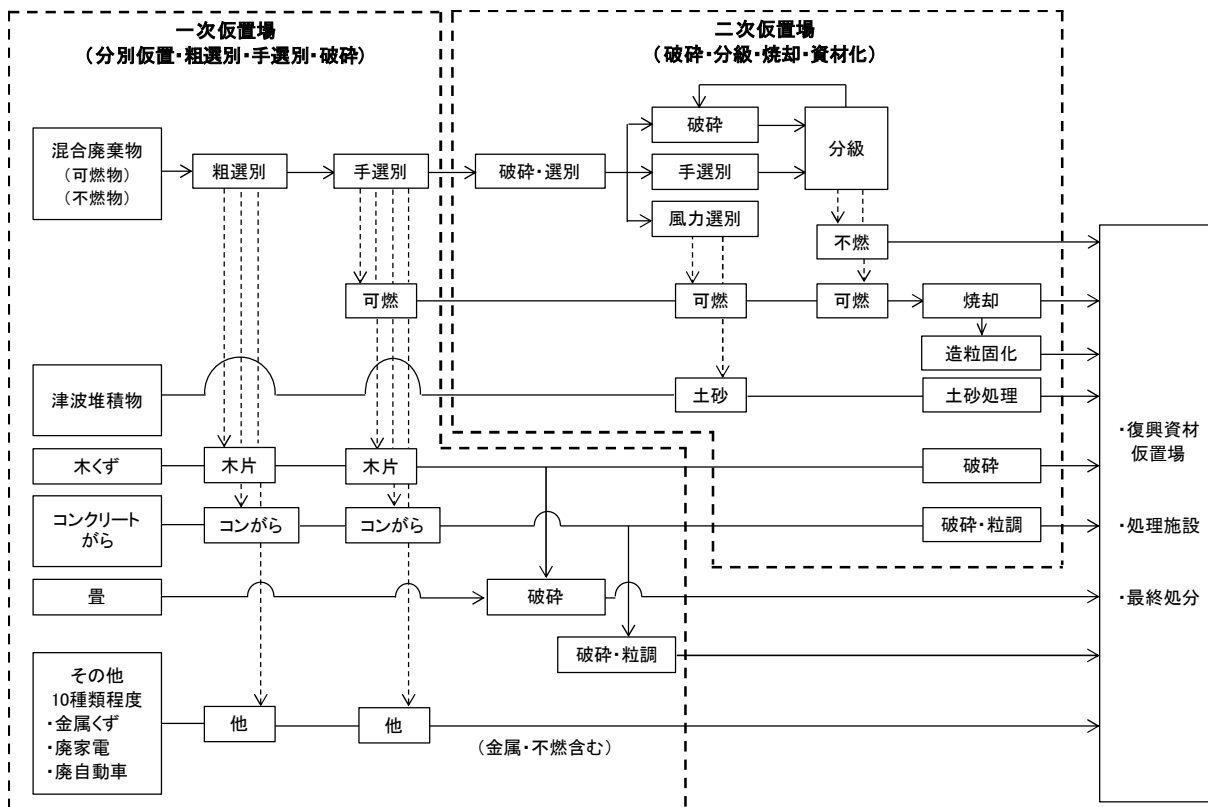
図表20 災害廃棄物の基本的な処理フロー
