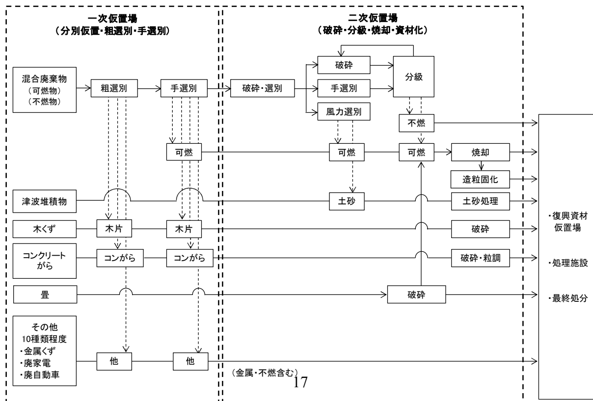
図表21 災害廃棄物の基本的な処理フロー（処理施設が設置できない場合）
