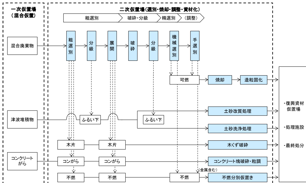
図表2.2 津波被害などにより廃棄物が混合した場合の処理フロー
